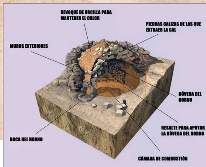
Esquema de funcionamiento de un horno de cal. http://hornodemontesa.blogspot.com.es
